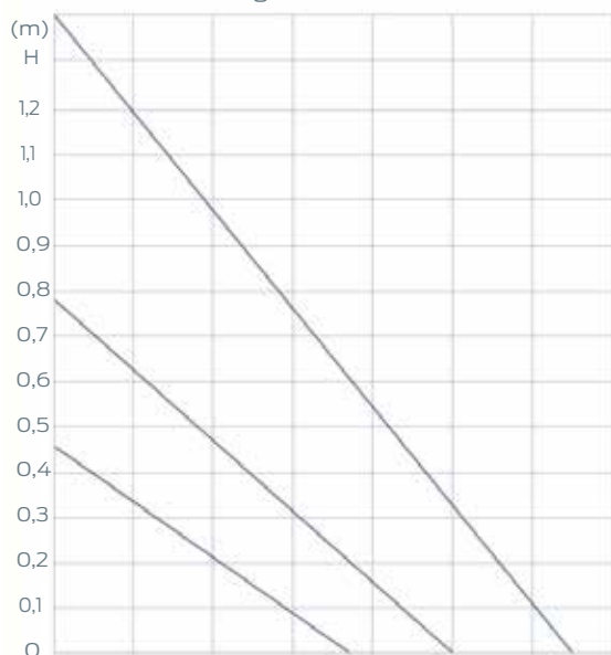
Karakteristikkurve go.future Z+
