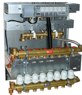
Neotherm Universalstativ
