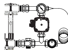
Montering till höger - anslutning från sidan
