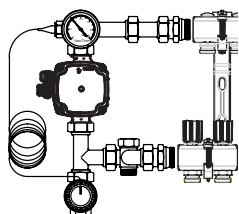
Montering till vänster - anslutning underifrån
