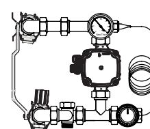
Montering vinklad framåt på Vänster sida - anslutning framifrån
