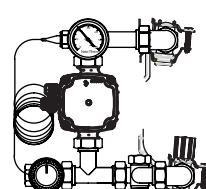
Montering vinklad bakåt på Vänster sida - anslutning bakifrån
