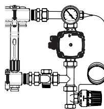
Montering till höger - anslutning underifrån
