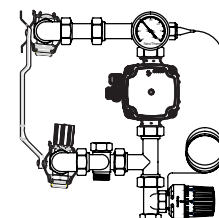
Montering vinklad framåt på Vänster sida - anslutning underifrån
