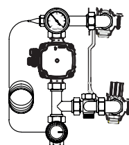
Montering vinklad bakåt på Vänster sida - anslutning underifrån
