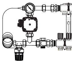
Montering till vänster - anslutning från sidan
