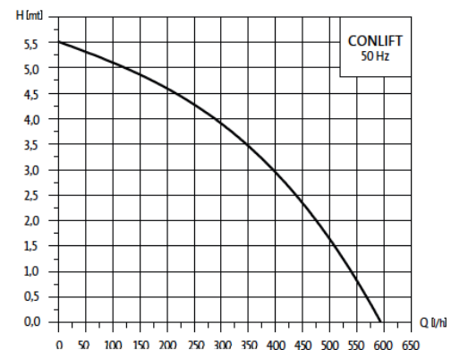
Kondensvattenpump CONLIFT - Ydelse
