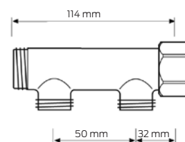
Rødgods fordelerrør 2 afgange
