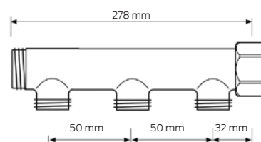
Rødgods fordelerrør 3 afgange
